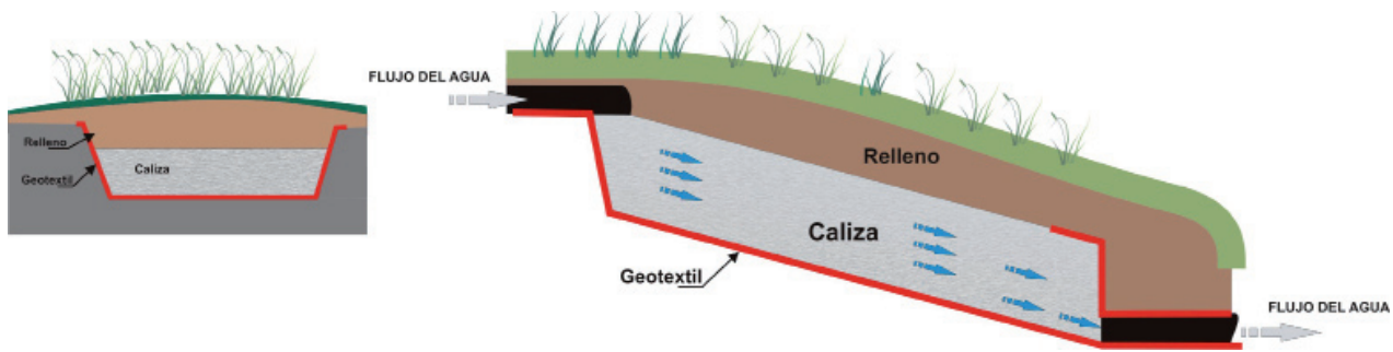
Figura 5.4 Esquema de un ALD
