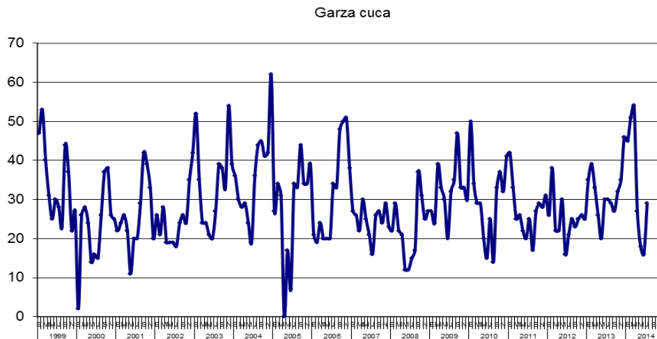
Figura 9. Abundancia de Garza cuca desde enero de 1999 a julio de 2014.
