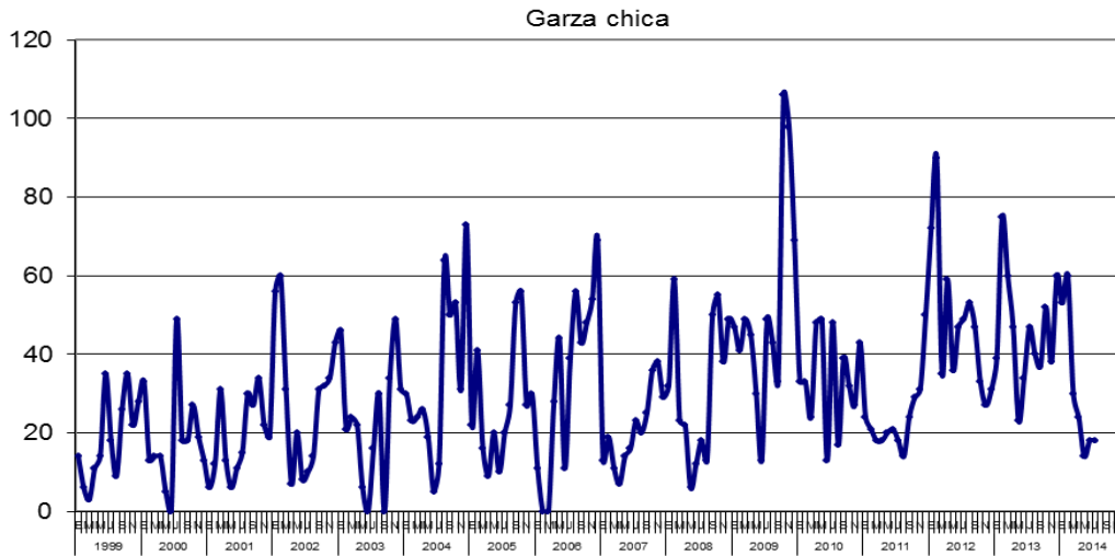
Figura 8. Abundancia de Garza chica desde enero de 1999 a julio de 2014.
