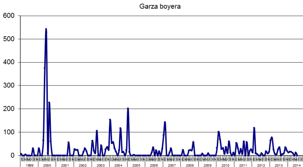
Figura 7. Abundancia de Garza boyera desde enero de 1999 a julio de 2014.
