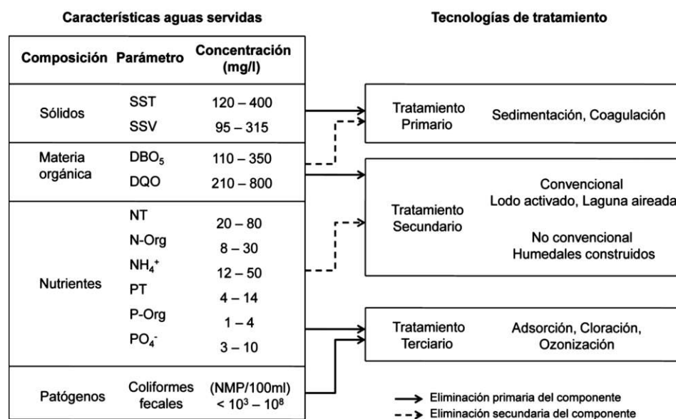
Figura 1. Características y tecnologías utilizadas en el tratamiento de aguas servidas. Fuente. Morales et. Al., 2013.
